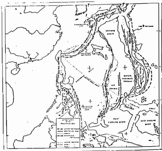
第一圖 遠東花綵列島中臺灣弧之位置 (HESS原圖)
