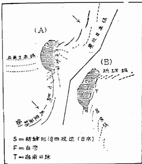
第二圖 臺灣與日本中部之紡錘形地塊之比較 (富田氏原圖)
