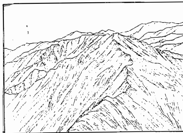
由玉山主山山頂北望玉山北山，其東坡為一標準之傾斜坡（dip slope）。玉山北山最高峰附近有臺灣最高之氣象觀測所。
