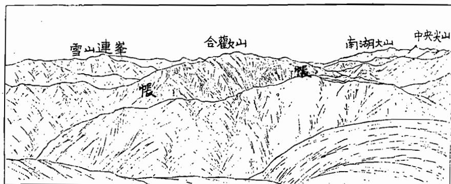
北合歡山之全景。右側遠方有中央尖山與其背後之南湖大山。左側遠處者為雪山之連峰。
