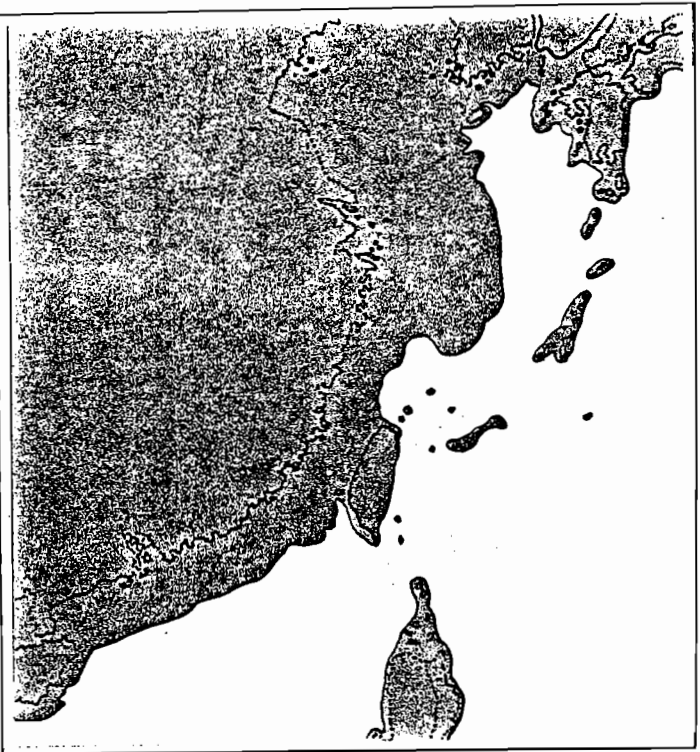
在一百多萬年前的冰河期，海水面曾下降一百多公尺，顯露出臺灣與大陸相連結的情形。
