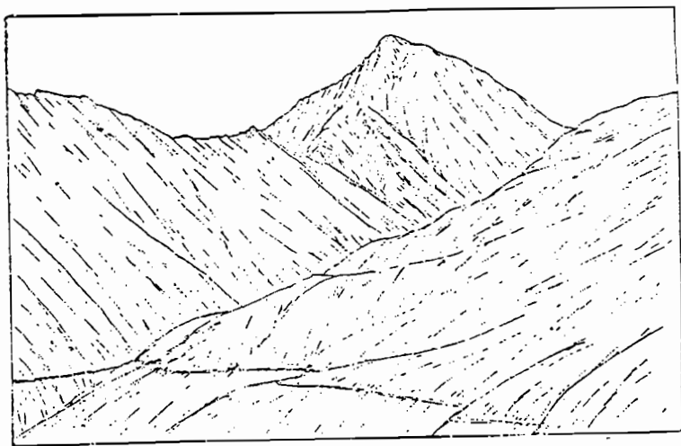
秀姑巒山爲脊梁山脈之一雄峯，海拔三八三三公尺，前面之山路爲八通關通玉里之「八通關越」登山路。
