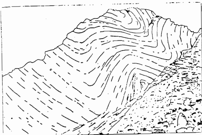
玉山主山的複雜褶皺（市村氏原圖）
