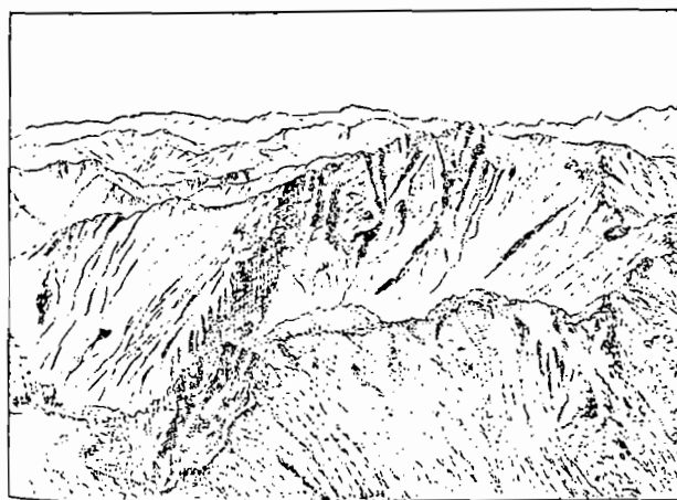
由玉山主山山頂南望玉山南山與南玉山一帶之羣峰
